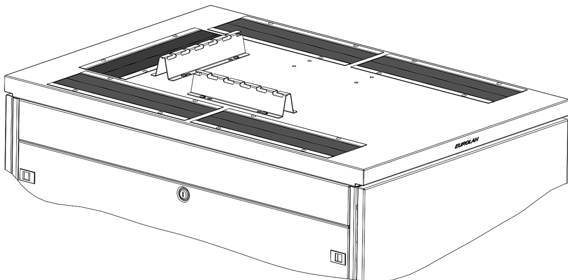
Рисунок 1. Установка набора для крепления лотков к крыше шкафа
