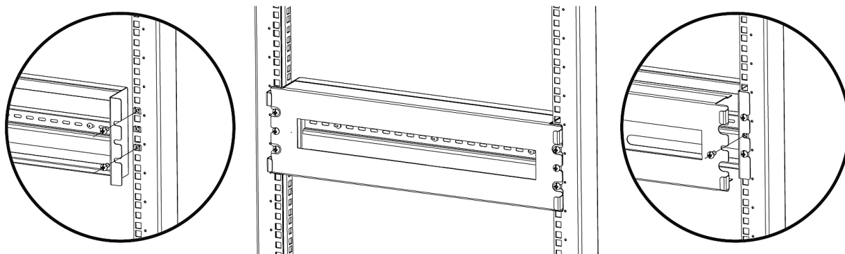
Рисунок 1. Установка панели 19" с DIN-рейкой
