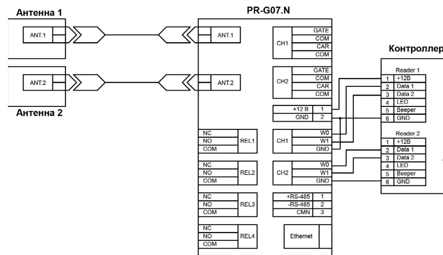
Рисунок 14. Интерфейс Wiegand
