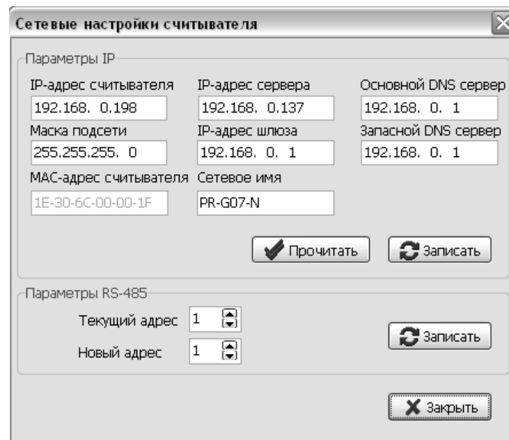
Рисунок 25. Окно настройки адресов считывателя
