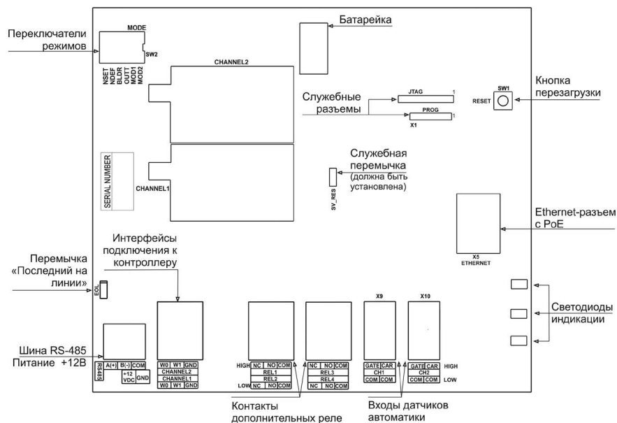
Рисунок 1. Схема расположения основных элементов считывателя PR-G07.N
