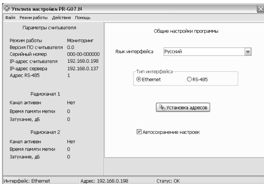
Рисунок 24. Окно общих настроек
