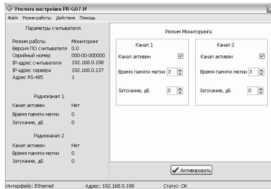
Рисунок 22. Стартовое окно утилиты
