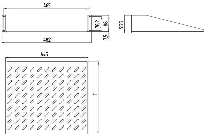
Технический эскиз
