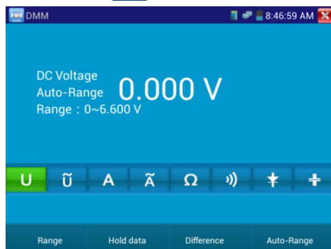
Рис. 3.3.17-1 Цифровой мультиметр
