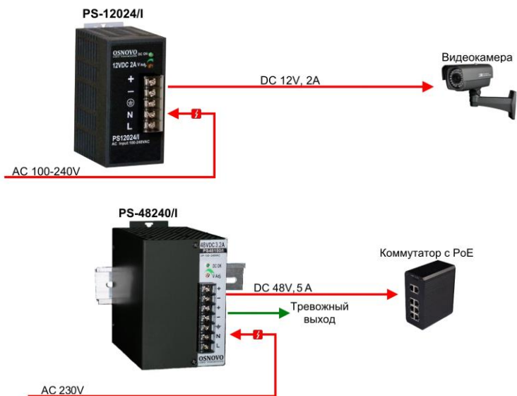
Рис. 3 Подключения блоков питания PS-12024/I, PS-48048/I PS-48150/I, PS-48240/I
