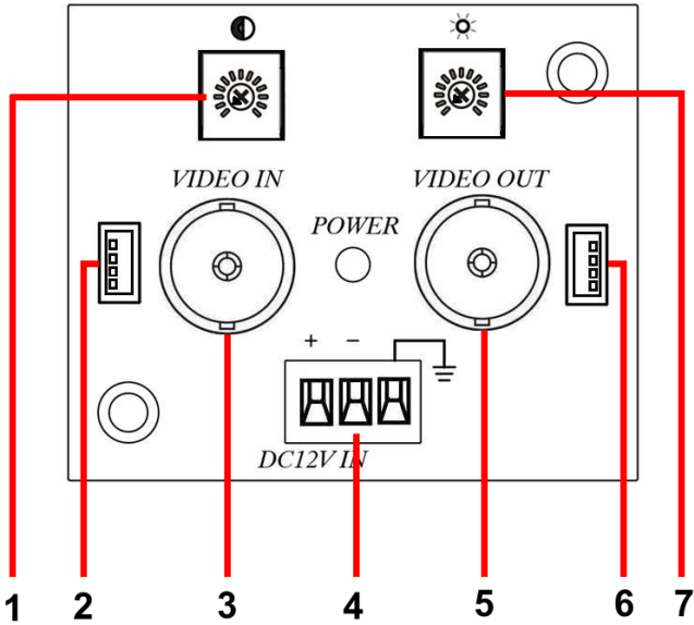
Рис. 2 Усилитель CA101HD, разъемы и регуляторы
