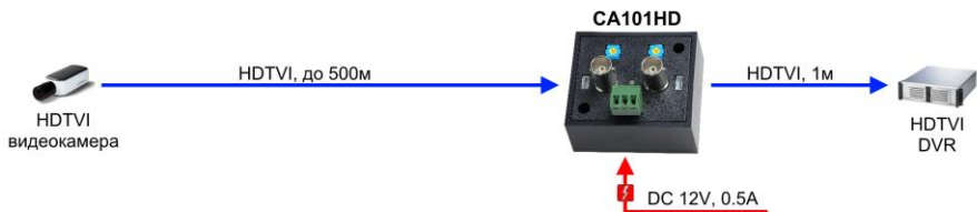
Рис.3 Схема подключения усилителя CA101HD на примере работы с HDTV-видеокамерами
