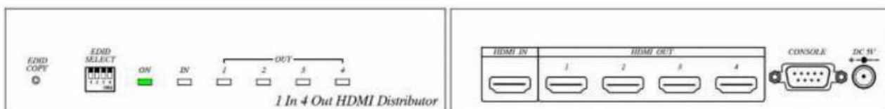
Рис. 3 Элементы передней и задней панелей HD04-4K
