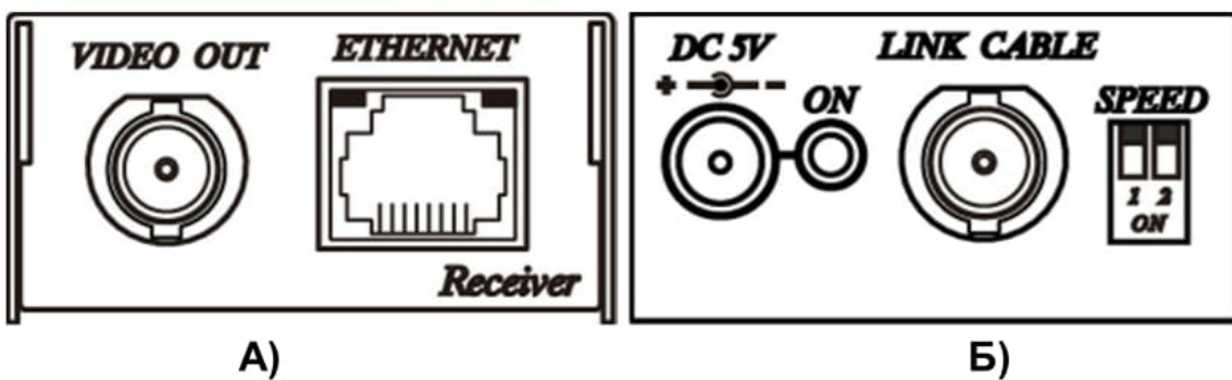
Рис.2 Разъемы и индикаторы передней (А) и задней (Б) панели
