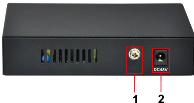
Рис. 3 Коммутатор SW-20500/MB(60W), разъемы и клеммы на задней панели
