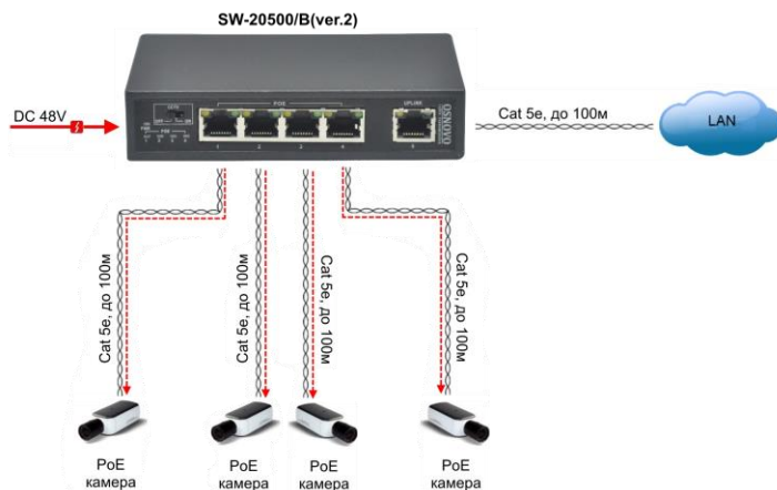
Рис.4 Типовая схема подключения коммутатора SW-20500/B(ver.2)
