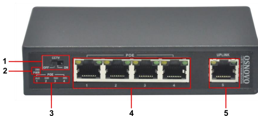
Рис. 2 Коммутатор SW-20500/B(ver.2), разъемы и индикаторы на передней панели
