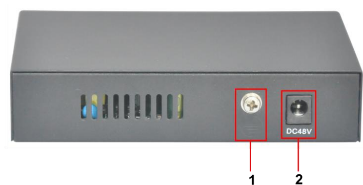
Рис. 3 Коммутатор SW-20500/B(ver.2), разъемы и клеммы на задней панели
