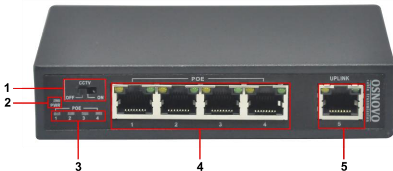
Рис. 2 Коммутатор SW-20500(без БП), разъемы и индикаторы на передней панели
