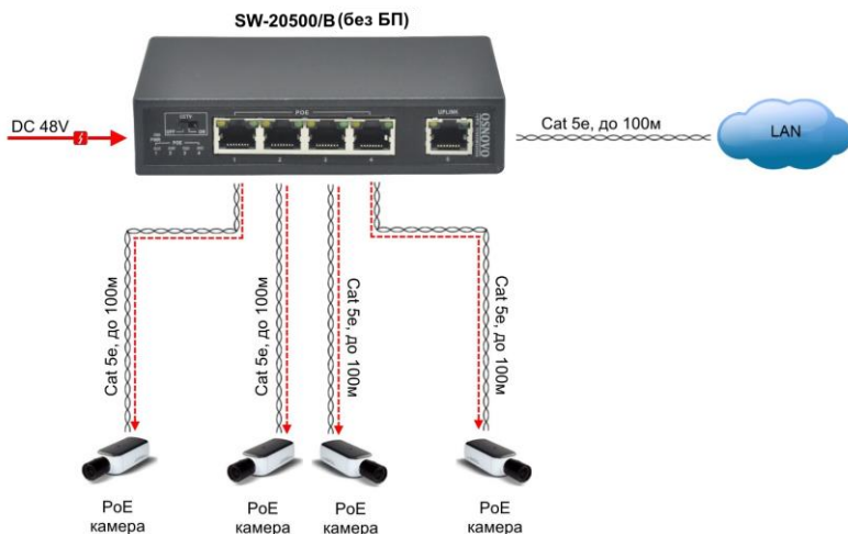
Рис.4 Типовая схема подключения коммутатора SW-20500(без БП)
