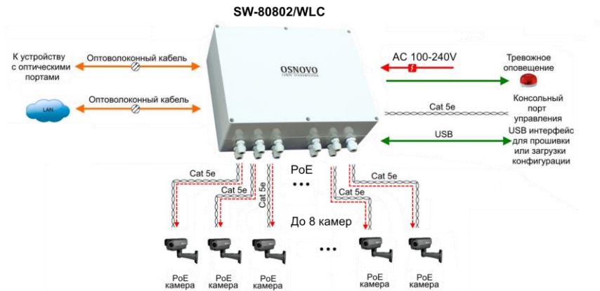
Рис.6 Типовая схема подключения уличного коммутатора SW-80802/WLC
