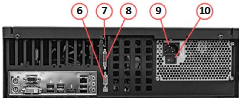
Рисунок 2. Задняя панель
